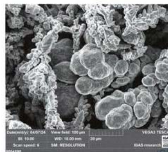
Fig. 4: 0004890 Cu powder. View field: 100 µm, scale: 20µm.
